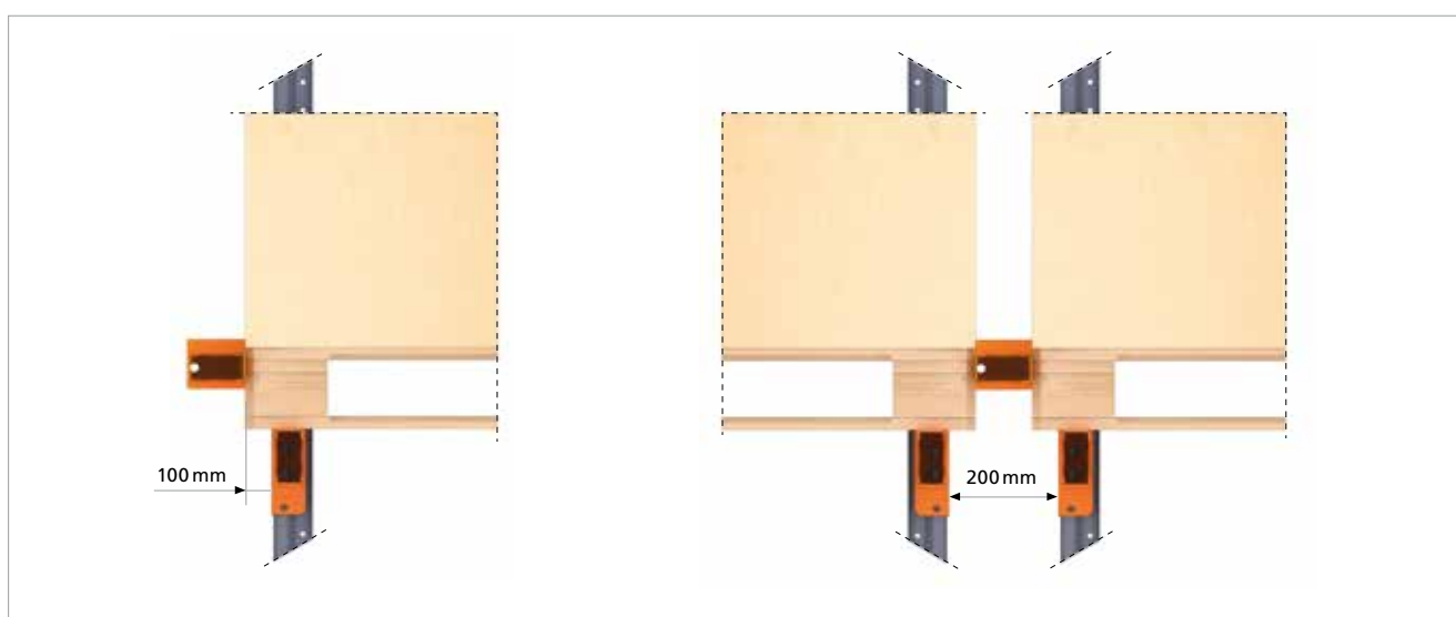
Alineación simple y doble con tope paleta
